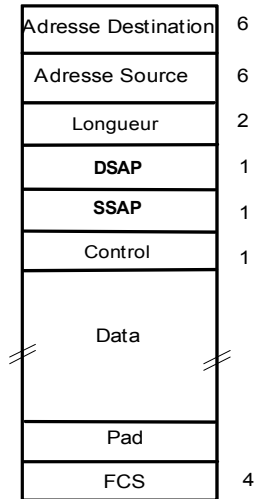
802.3 avec 802.2
