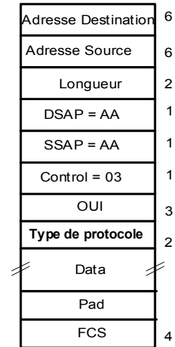
802.3 avec 802.2 SNAP
