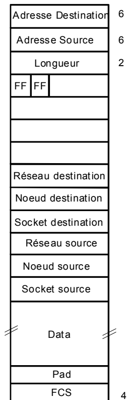
802.3 sans 802.2 (802.3 Raw)
